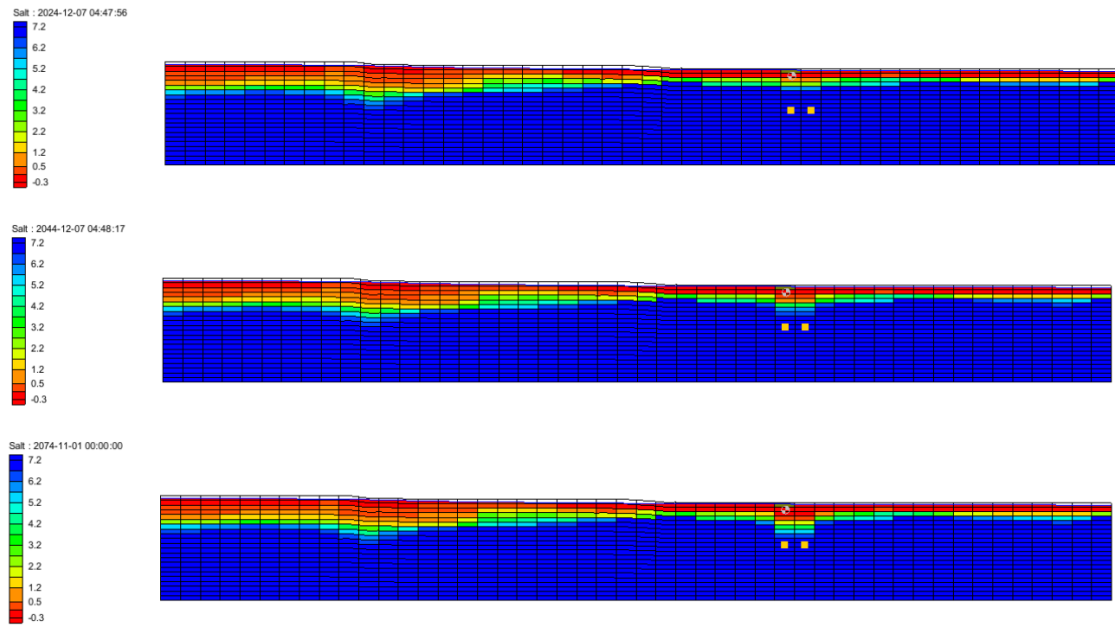
Figur 16: Sötvattenlinsens sänkning vid ett pumpflöde på 10 m³/(d·pump). Profilerna visar saltlinsen efter 10, 30 och 60 års pumpning från A till C i figur 10
