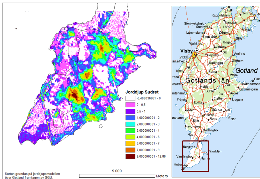
Figur 2: Jorddjup [m] samt delavrinningsområden på Sudret, södra Gotland. Skapad utifrån jorddjupsmodellen framtagna av SGU samt delavrinningsområden från SHMI.©SGU
