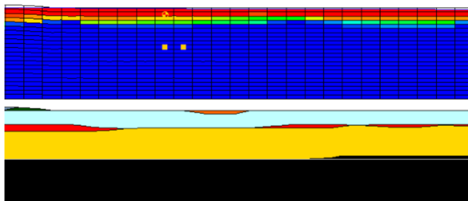
Figur 14: Salthalt [ \text{kg/m}^3 ] efter 2400 års simulering samt geologi i genomskärning från syd till norr (B till C i figur 10. Profilen sträcker sig från markytan cirka 12 m.ö.h ner till 150 m.u.h.
