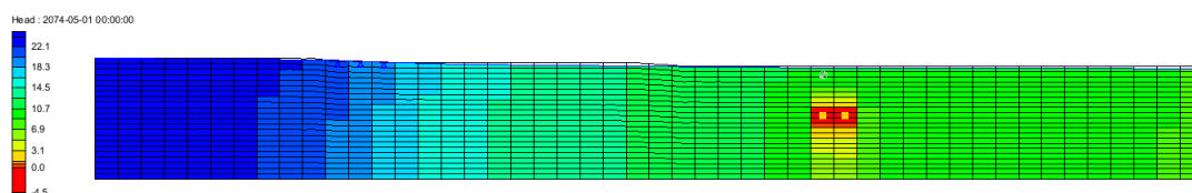
Figur 18: Hydraulisk potential över profilen från A till C i figur 10 i slutet av den sista pumppperioden vid ett pumpflöde på 10 \text{ m}^3/(\text{d}\cdot\text{pump}) .
