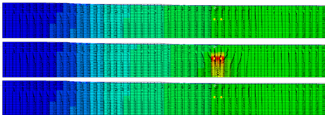
Figur 25: Grundvattnets flödesriktningar före-, under- och efter pumpning.
