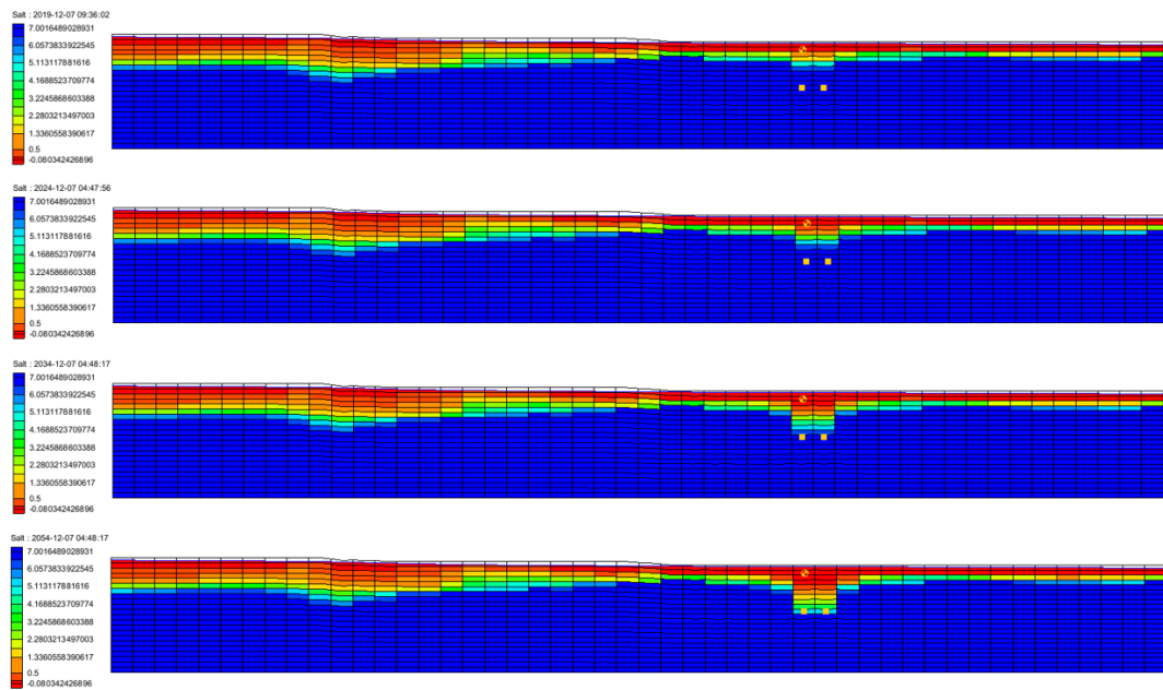
Figur 17: Sötvattenlinsens sänkning vid ett pumpflöde på 40 m³/(d·pump). Profilerna visar saltlinsen från A till C i figur 10 efter 5, 10, 20 och 40 års pumpning.
