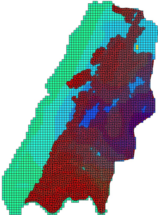
Figur 9: Gula prickar anger pumparnas position och rött område visar hur mörgelstråket sträcker sig över modellen.
