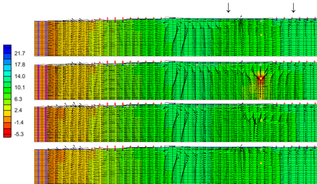
Figur 23: Grundvattnets flödesriktningar. Från toppbilden till bottenbilden:
