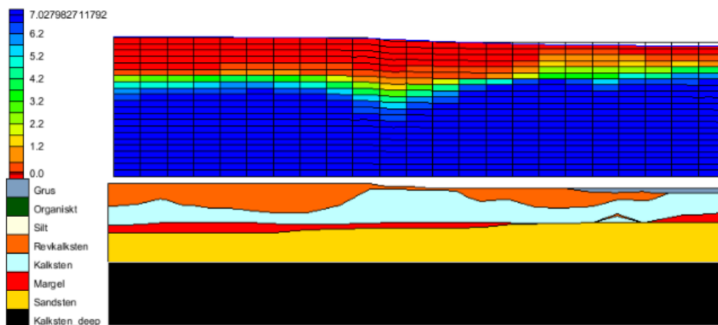
Figur 13: Salthalt [ \text{kg/m}^3 ] efter 2400 års simulering samt geologi i genomskärning från syd till norr (A till B i figur 10. Profilen sträcker sig från markytan cirka 24 m.ö.h ner till 150 m.u.h.
